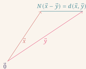
FIGURE 1 – Distance entre deux vecteurs \vec{x} et \vec{y}
