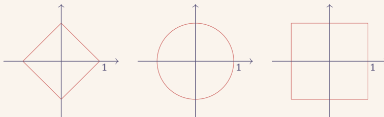
FIGURE 3 – Sphère de centre \vec{0} et de rayon 1 pour les normes 1, 2 et \infty de \mathbb{R}^2
