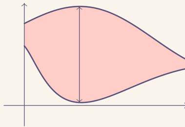
FIGURE 2 – Distance entre deux fonctions
